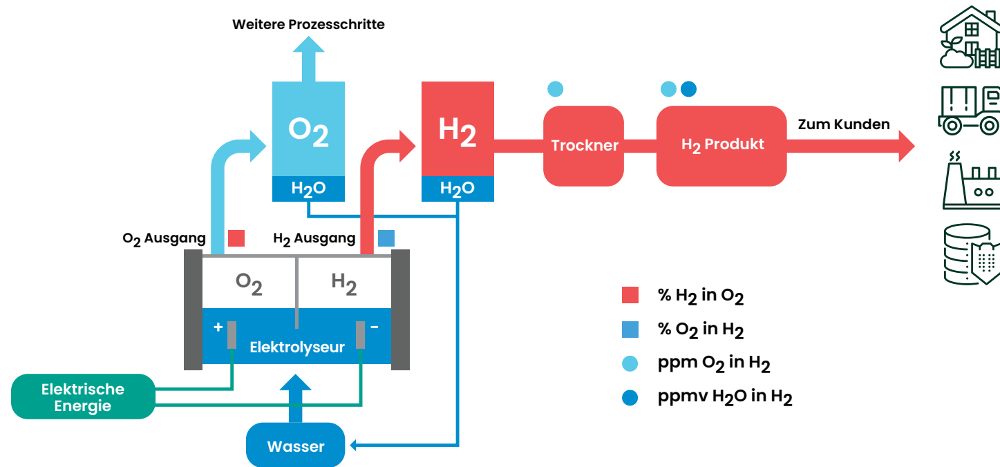
Typischer Elektrolyseprozess
